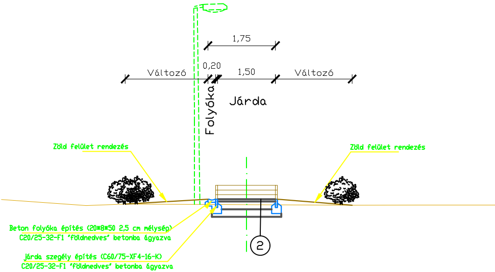
Mintakeresztmetszvény (M7) Kert utca - gyalogos járda és lépcső
